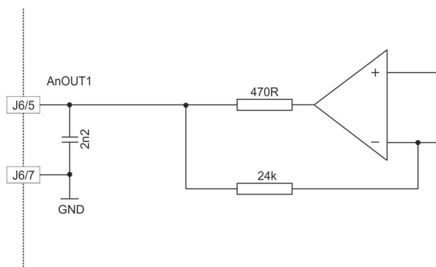
图 3-18 AnOUT1 的连接 (AnOUT2 的连接方式类似)
