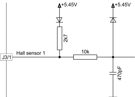
图 3-6 霍尔传感器 1 输入端的连接（霍尔传感器 2 和 3 的连接方式类似）
