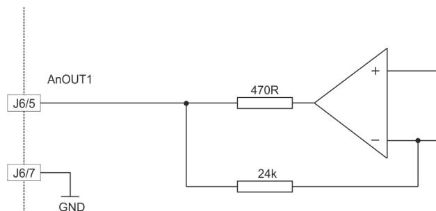
图 3-15 AnOUT1 的连接 (AnOUT2 的连接方式类似)
