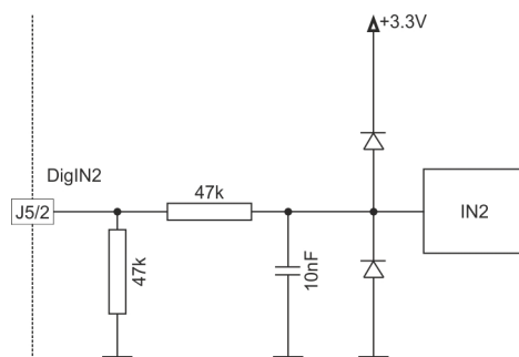
图 3-9 DigIN2 的连接
