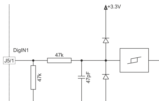
图 3-8 DigIN1 的连接
