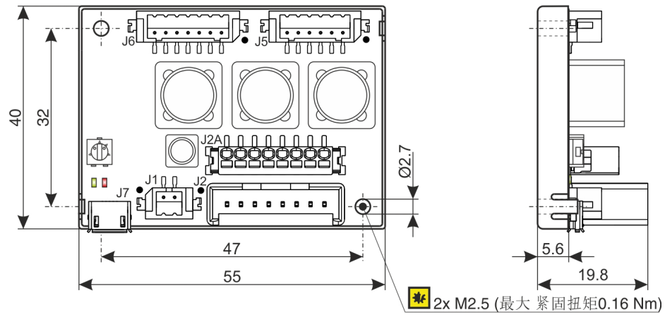
图 2-2 尺寸图 [mm]
